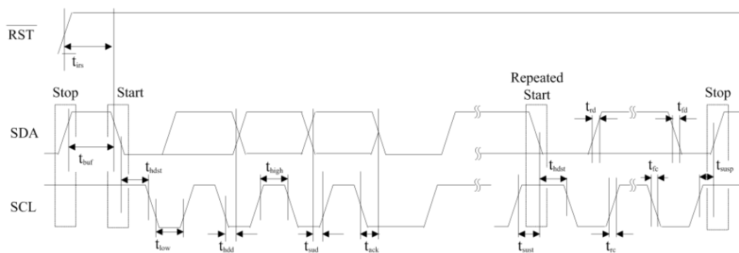
图 6. I 2 C 模式时序
