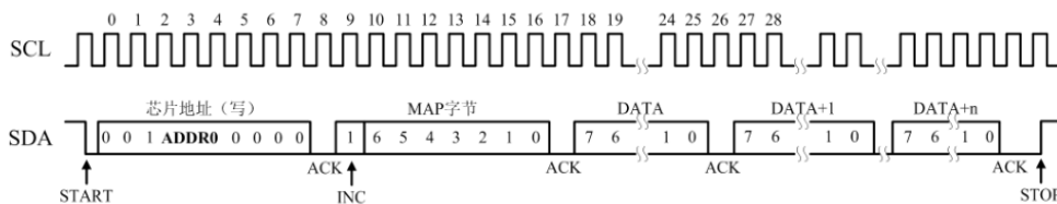
图四、控制端口时序（I 2 C 从模式写）
