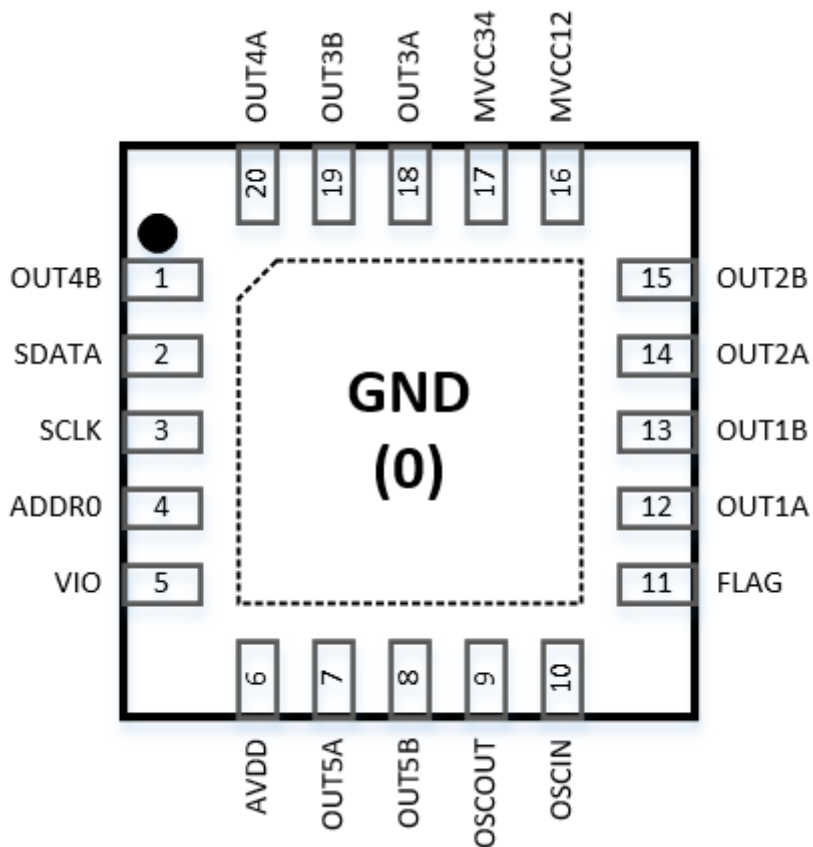
图二、SC7510 管脚图 (Top View)
