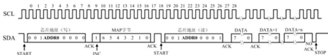
图五、控制端口时序（I 2 C 从模式读）
