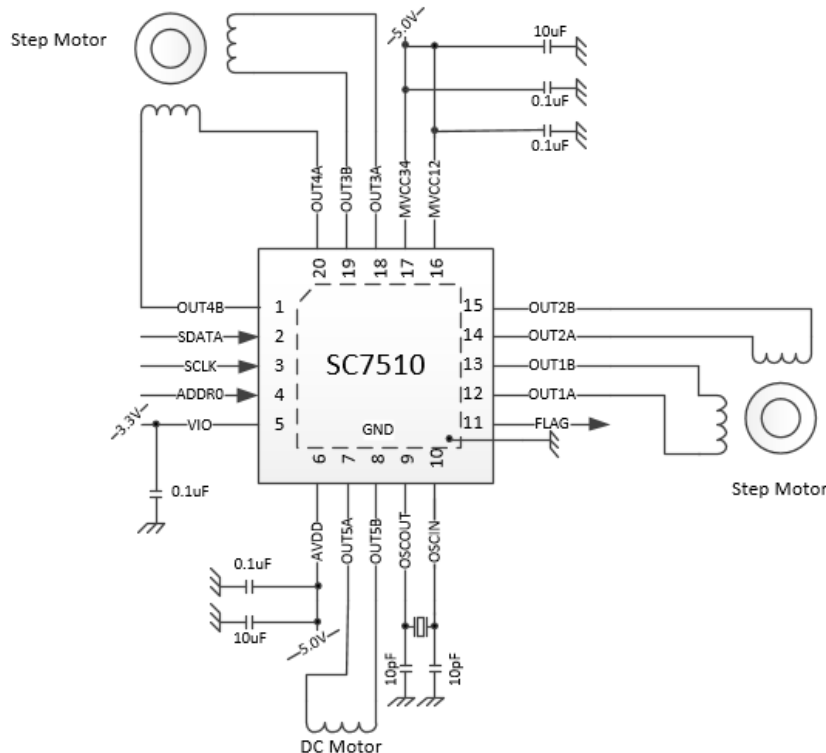
图一、典型应用图
