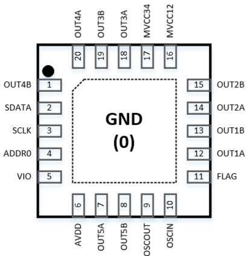
图二、SC7520 管脚图 (Top View)
