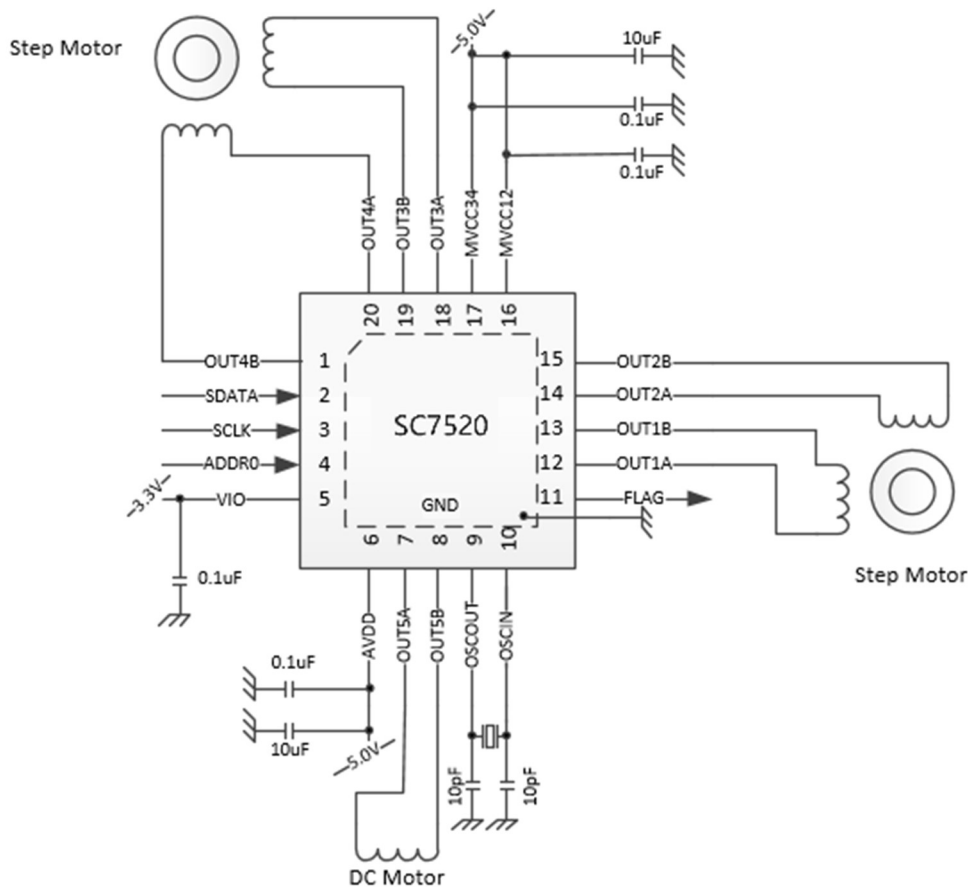
图一、典型应用图
