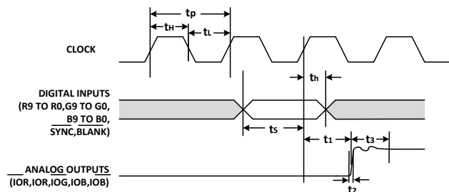
Figure12. Video Data Input/Output
